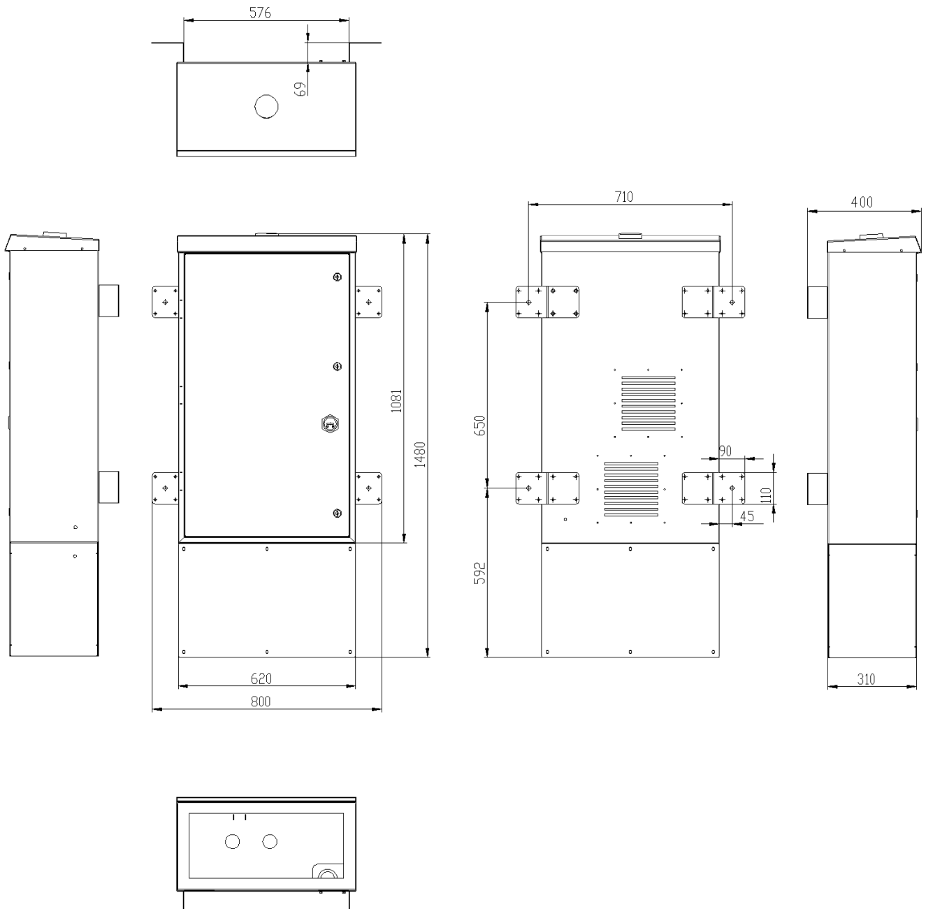
Рисунок 1 – Габаритные и установочные размеры при креплении АПВ на стене
