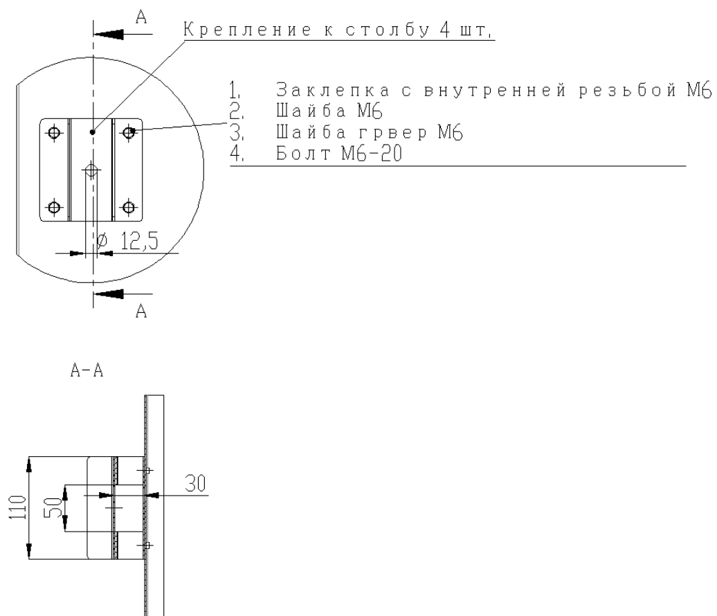
Рисунок 4 – Крепление АПВ на опоре
