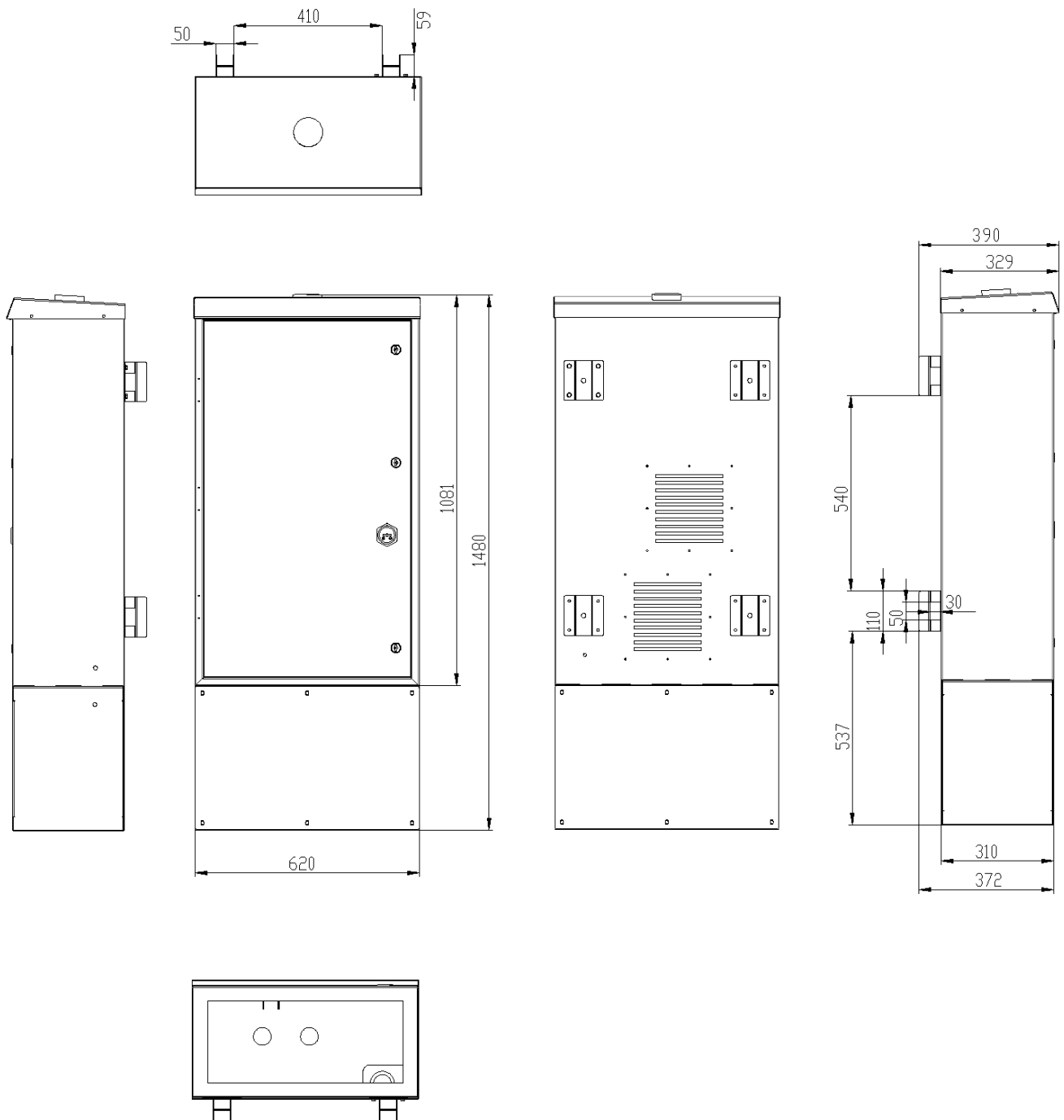
Рисунок 2 – Габаритные и установочные размеры при креплении АПВ на опоре
