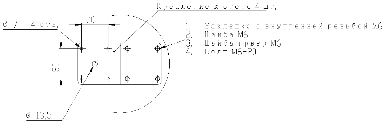
Рисунок 3 – Крепление АПВ на стене
